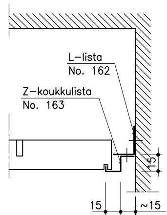
Säädettävä
