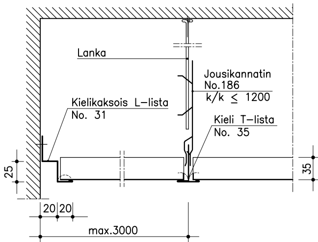
RAKENNEDETALJIT ESITE 6.1
