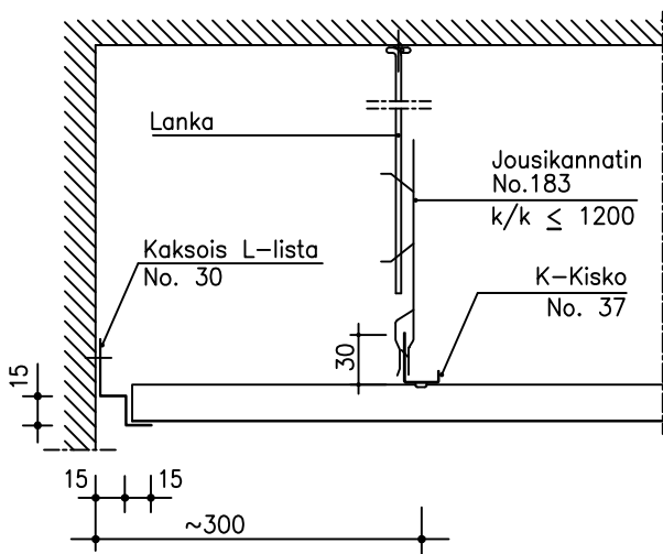
RAKENNEDETALJIT ESITE 6.1
