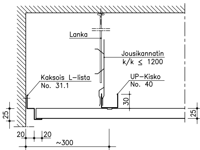
RAKENNEDETALJIT ESITE 6.1
